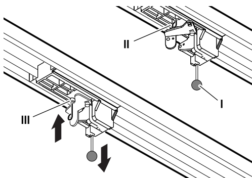
Fig. 9: Déverrouillage et verrouillage de l'entraînement
