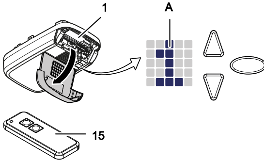
Ábra 4: Kezelőelemek
