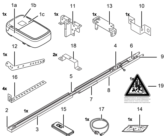
III. 2: Produktoversikt - Enkeltodeler
